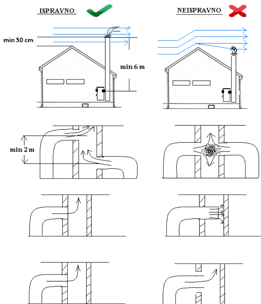
Slika 1. POSTAVLJANJE PEĆI
